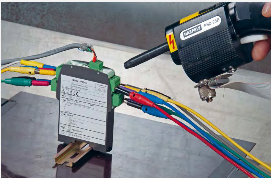
Prüfung eines SINEAX V604s auf Störfestigkeit gegen elektrostatische Entladungen (ESD)
